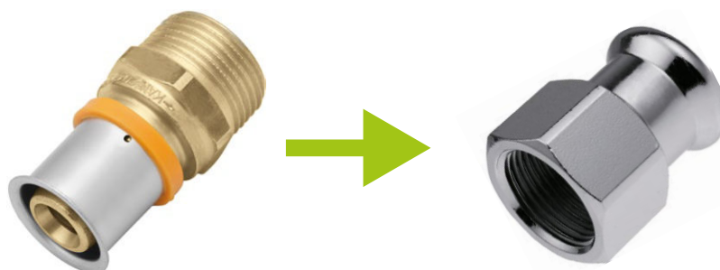
KAN-therm Inox 304 sistēmu tērauda elementu savienošana ar misiņa elementiem
