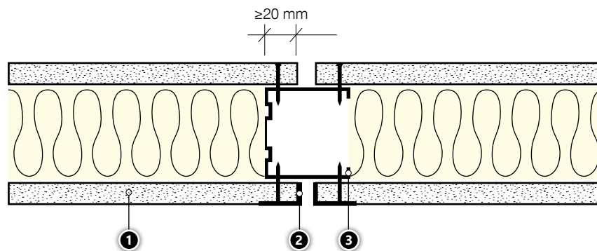
Att. 42. Atvērta sprauga
