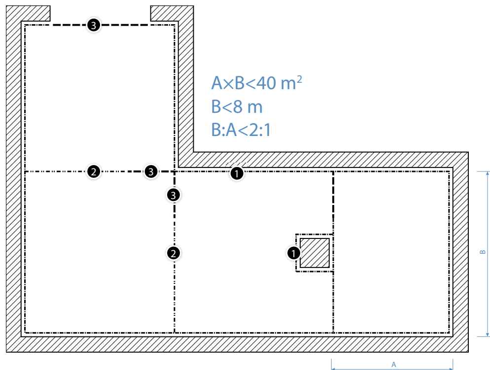
Att. 18. Kompensācijas šuves izveide starp grīdas apkures plāksnēm
