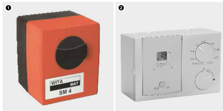
Att. 52. KAN-therm centrālās sajaukšanas sistēmas vadības elementi (SM4 pievads (1) un laikapstākļu regulators (2))
