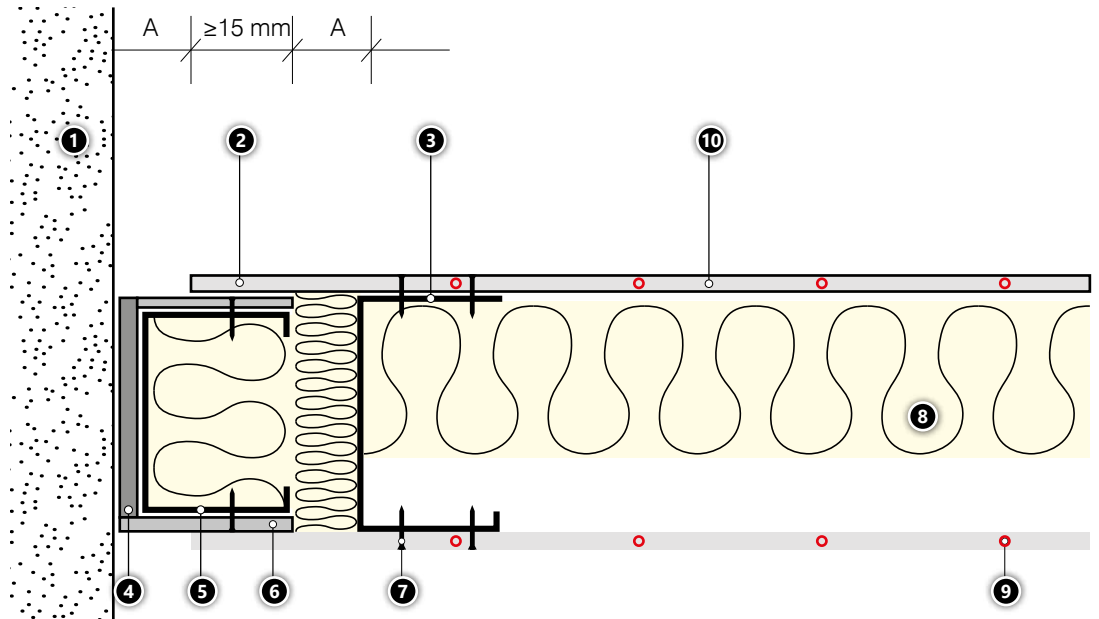
Att. 41. Slidošais savienojums ar sienu.
