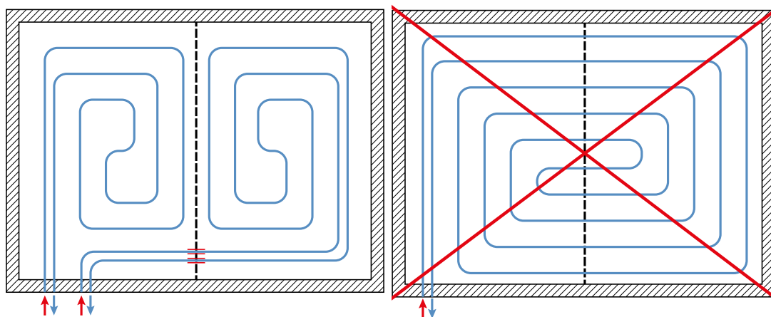
Att. 19. Pareizs un nepareizs apkures laukumu sadalījums ar kompensācijas šuvi
