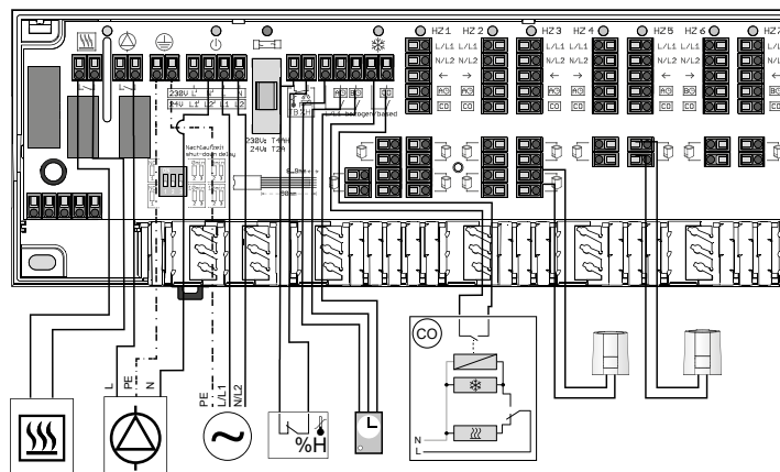
Att. 72. Elektriskā bloka Basic+ 230 V vai 24 V ar sūkņa un katla moduli un perifērājam ierīcēm konfigurācija.
