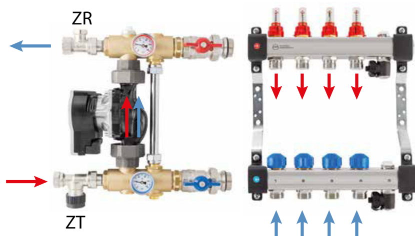
Att. 58. Fiksētas vērtības sūkņu grupa ar UFST kolektoru — plūsmas virzieni.
