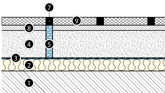
Att. 16. Kompensācijas šuves izveide uz akmens seguma
