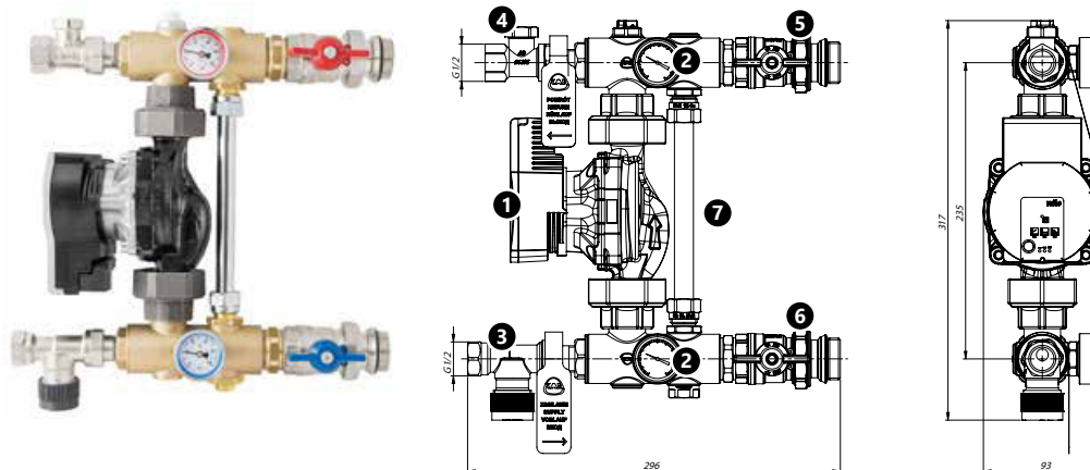
Att. 54. KAN-therm sūkņu grupas konstrukcija
