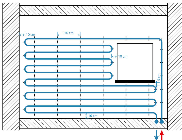
Att. 34. Uzstādīšanas atstatumi sienu apsildē
