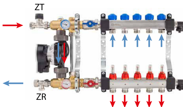
Att. 57. Kolektors, kas aprīkots ar USFP, ar maisīšanas vienību sistēmu—plūsmas virzieni
