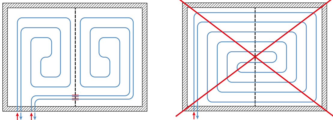
Att. 19. Pareizs un nepareizs apkures laukumu sadalījums ar kompensācijas šuvi
