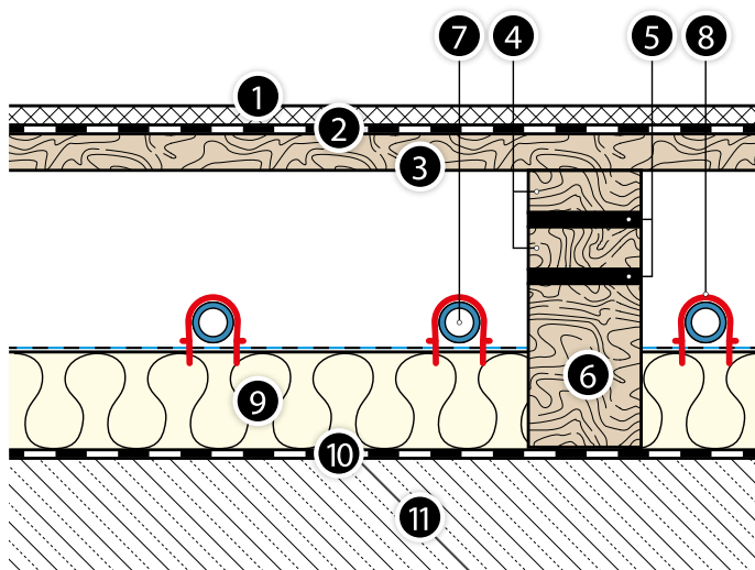
Att. 32. Vienmērīgi elastīgas sporta grīdas šķersgriezums, no KAN-therm Tacker grīdas apsildes sistēmas elementiem
