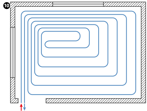
Att. 9. Grīdas apkures/dzesēšanas cilpa, izmantojot kombinētu savienošanas tehniku: dubultais likumveida savienojums. Att. 10. Grīdas apkures/dzesēšanas cilpa spirālveida izkārtojumā, ar malu zonu uz vienas cilpas, kas ieklāta gar ārējām sienām vai virsmām ar lielu stiklojumu.
