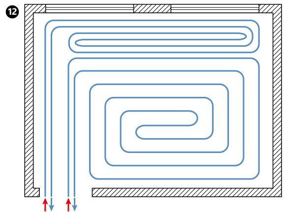
Att. 11. Grīdas apkures/dzesēšanas cilpa likumveida izkārtojumā, ar malu zonu uz vienas cilpas, kas ieklāts gar ārējām sienām vai virsmām ar lielu stiklojumu a laukumug. Att. 12. Grīdas apkures/dzesēšanas cilpa spirālveida izkārtojumā, ar malu zonu uz atsevišķas cilpas, kas ieklāta gar ārējām sienām vai virsmām ar lielu stiklojumu a laukumu.
