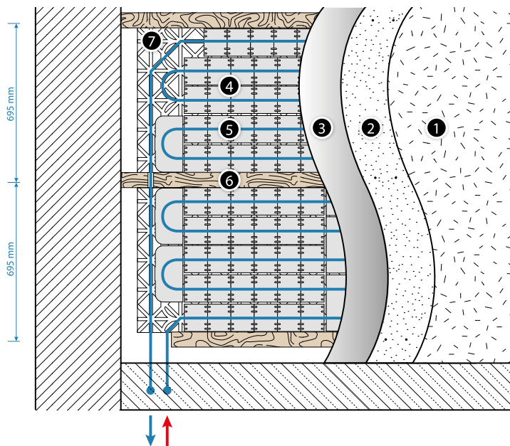
Att. 37. KAN-therm TBS sienas apsildes sistēmas šķēsgriezums.
