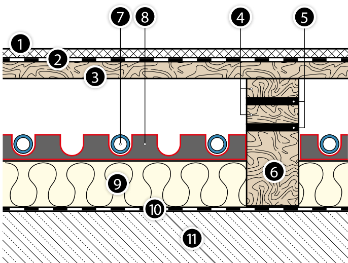
Att. 33. Vienmērīgi elastīgas sporta grīdas šķersgriezums, no KAN-therm Rail grīdas apsildes sistēmas elementiem.
