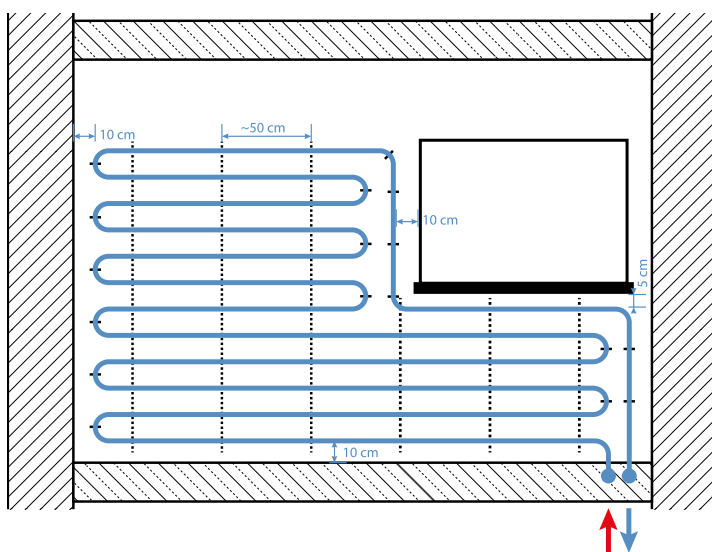
Att. 34. Uzstādīšanas atstatumi sienu apsildē
