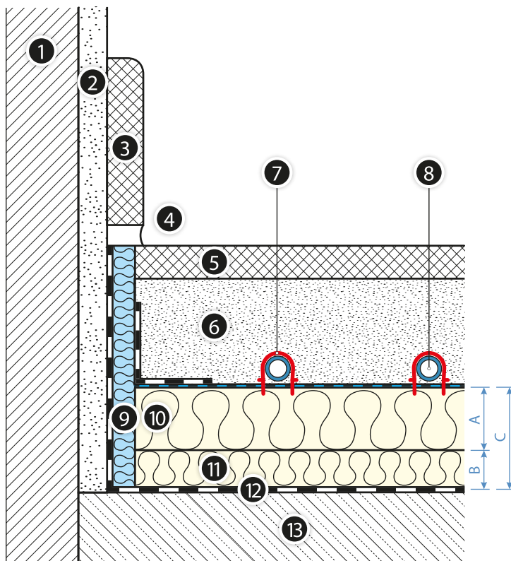
Att. 23. Sildītājs ar KAN-therm Tacker Sistēmas plāksni un papildu izolāciju un hidroizolāciju uz griestiem, kas atrodas saskarē ar grunti
