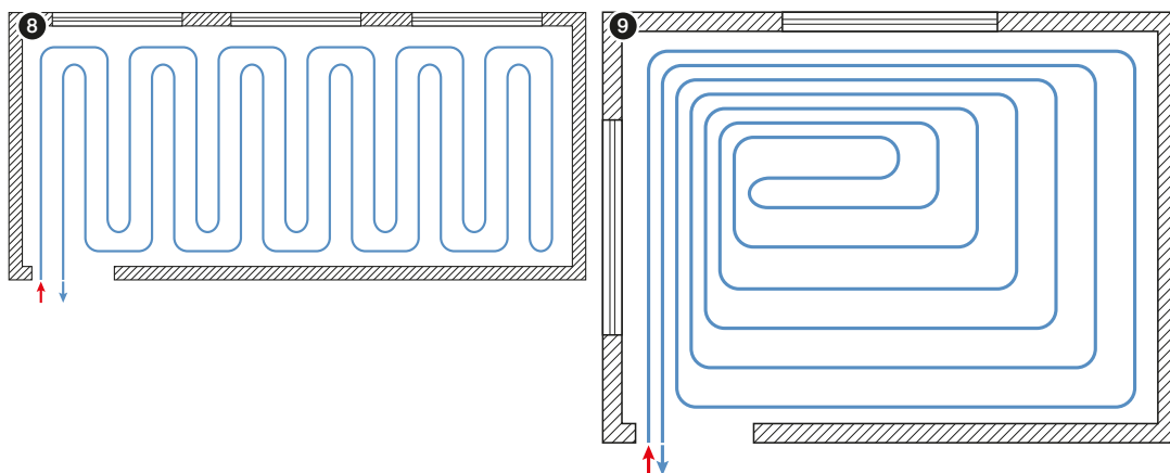
Att. 8. Grīdas apkures/dzesēšanas spirāle, izmantojot kombinētu savienošanas tehniku: dubultais līkumveida savienojums.
