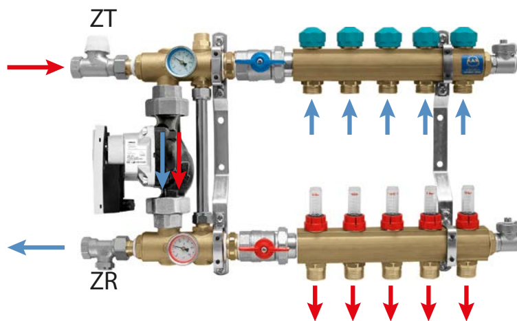
Att. 60. Sadalītājs ar sajaukšanas sistēmu 77E (vai 73E) – plūsmas virzieni
