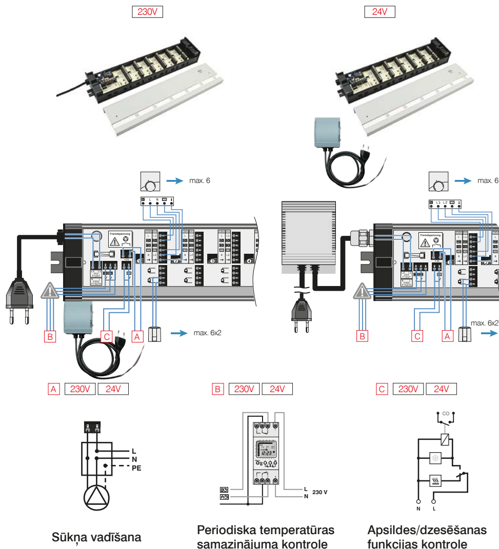
Att. 71. Basic apsildes/dzesēšanas spaiļu bloka 230V/24V konfigurācija ar sūkņa moduli
