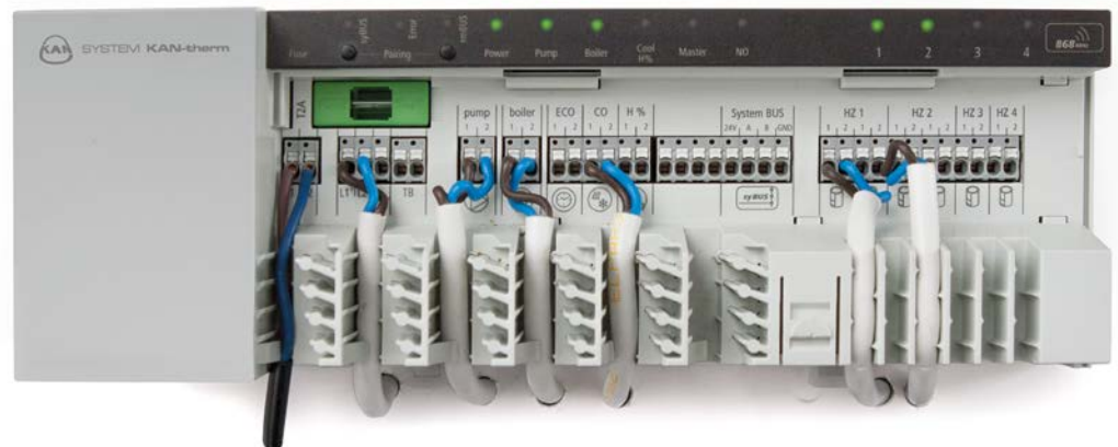
Att. 74. Skaidrs spaiļu bloka darbības stāvokļa attēlojums, vienkārša un droša pievadu un ārējo ierīču pieslēgšana.
