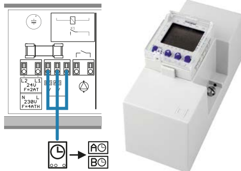
Att. 76. Pulksteņa pieslēgšanas shēma Basic spaiļu blokam
