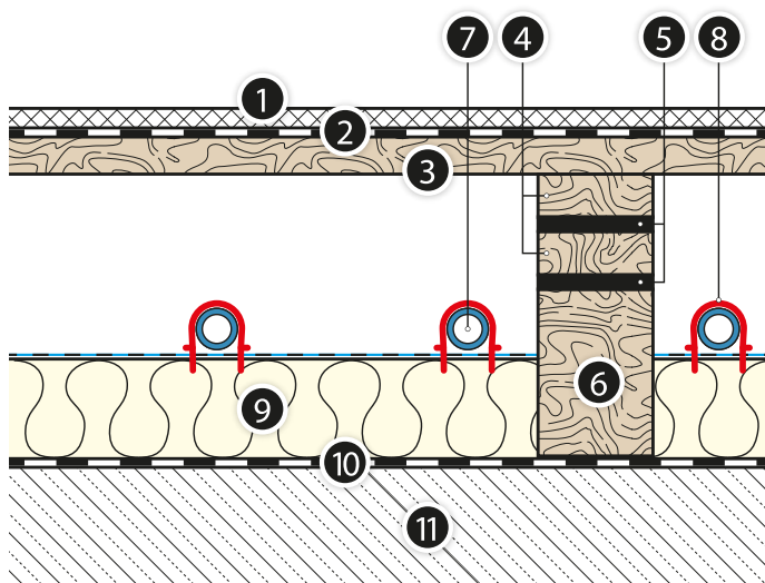
Att. 37. Vienmērīgi elastīgas sporta grīdas šķersgriezums, no KAN-therm Tacker grīdas apsildes sistēmas elementiem
