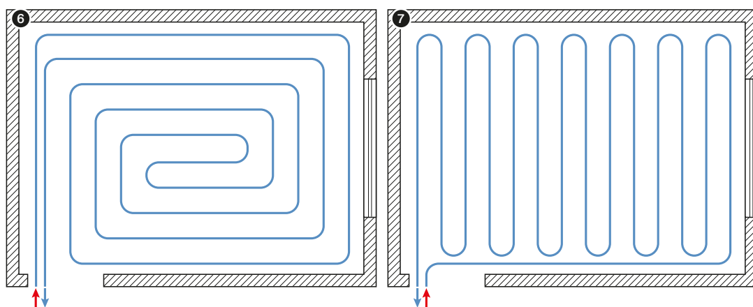
Att. 6. Grīdas apkures/dzesēšanas spirāle spirālveida izkārtojumā.
