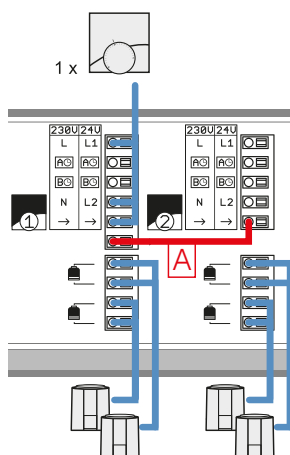
Att. 69. 3 vai 4 pievadu pieslēgums ar termoregulāciju
