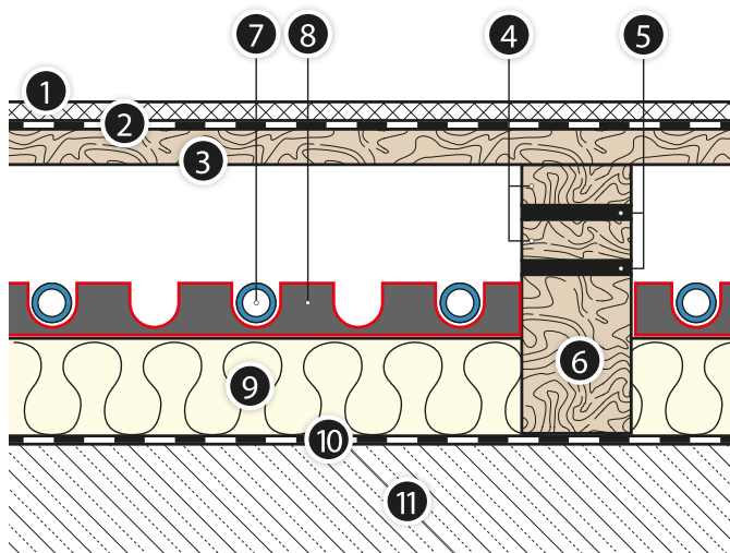
Att. 38. Vienmērīgi elastīgas sporta grīdas šķersgriezums, no KAN-therm Rail grīdas apsildes sistēmas elementiem
