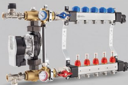
Kolektori ar plūsmas mērītājiem un ar servomotoriem aprīkoti vārstiem kā arī sajaukšanas mezglu ar cirkulācijas sūkni - sērija USFP
