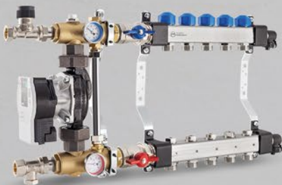
Kolektori ar regulējošajiem vārstiem un servopiedziņu vārstiem kā arī sajaukšanas mezglu ar cirkulācijas sūkni - sērija USVP
