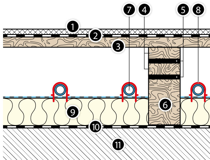
Att. 31. Vienmērīgi elastīgas sporta grīdas šķersgriezums, no KAN-therm Tacker grīdas apsildes sistēmas elementiem
