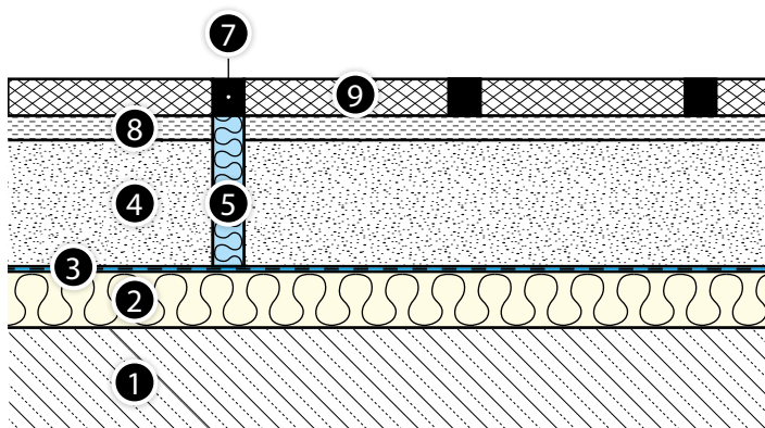
Att. 15. Kompensācijas šuves izveide uz akmens seguma
