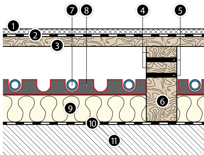
Att. 32. Vienmērīgi elastīgas sporta grīdas šķersgriezums, no KAN-therm Rail grīdas apsildes sistēmas elementiem.
